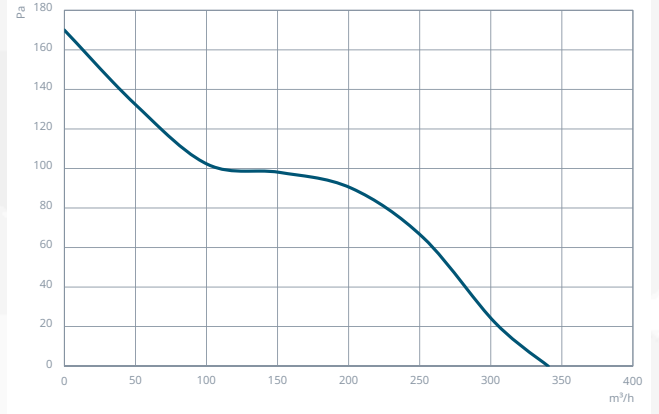
NMFF 125
