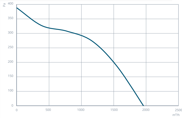
NMFF 315
