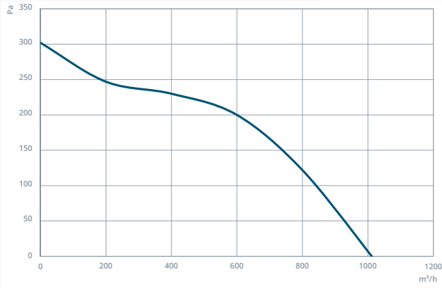
NMFF 200
