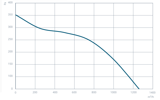
NMFF 250
