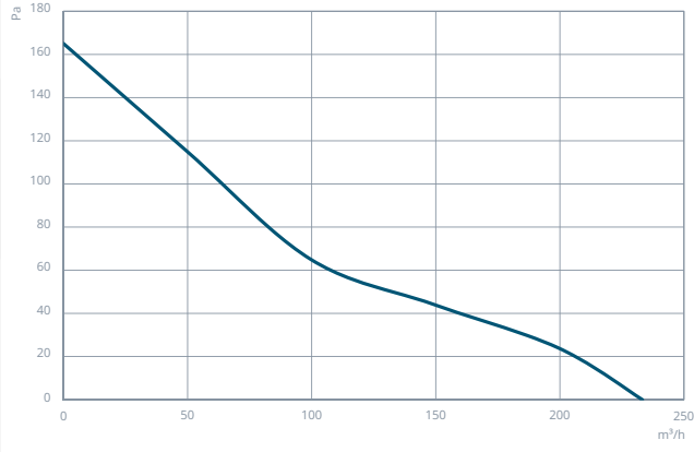
NMFF 100
