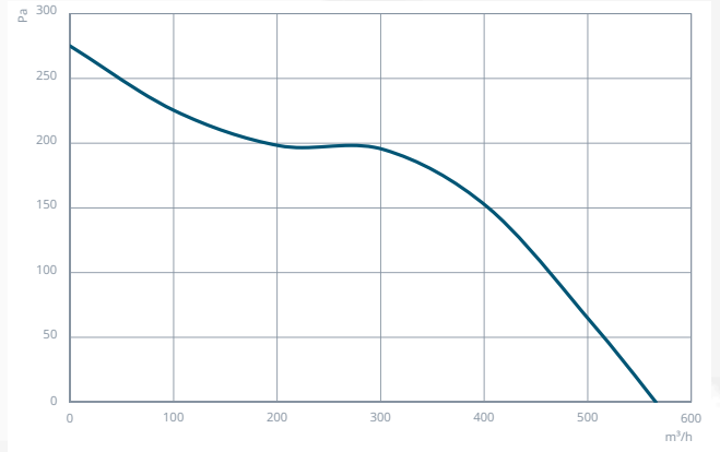
NMFF 160
