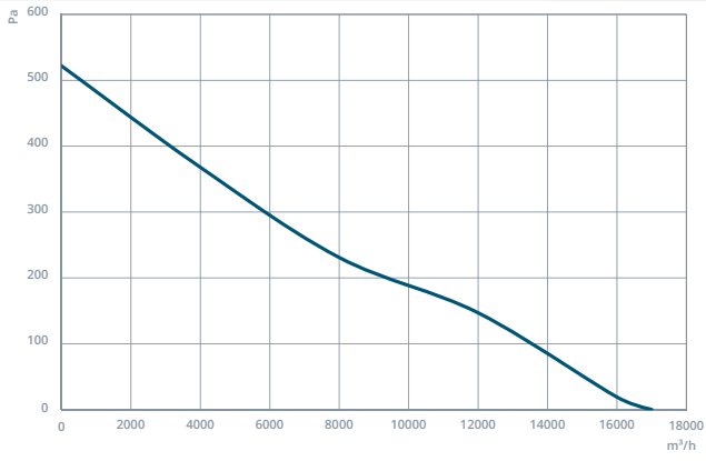
NDTF-SM 710-5-30
