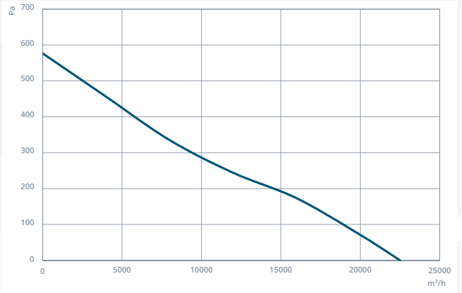
NDTF-SM 800-5-30
