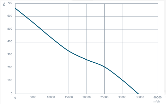
NDTF-SM 900-5-35
