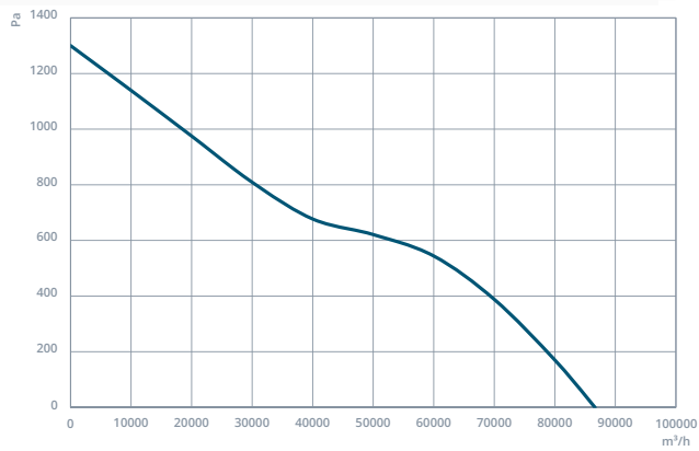
NDTF-DM 1120
