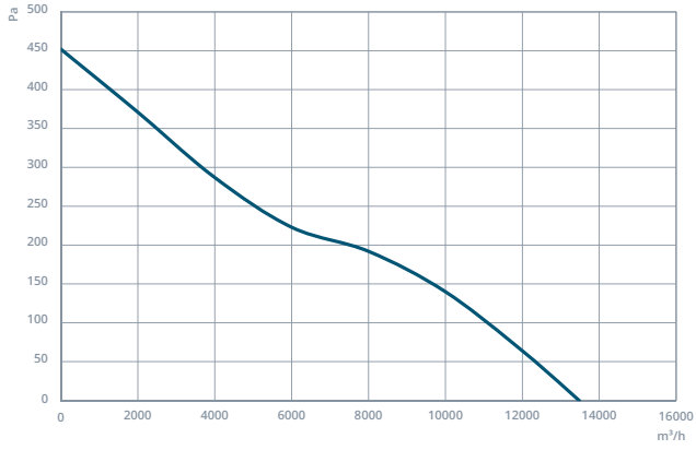
NDTF-DM 630
