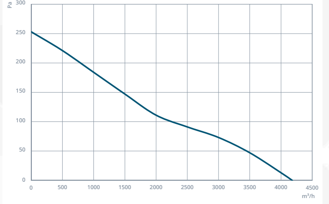
NDTF-DM 450
