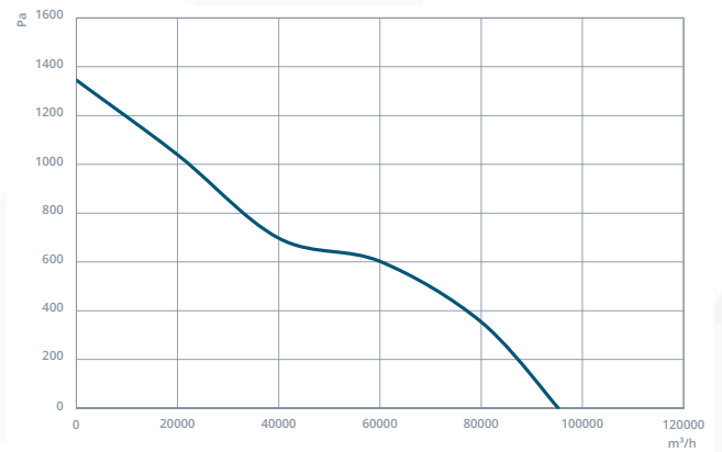
NDTF-DM 1120
