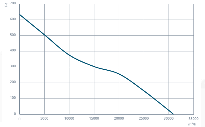
NDTF-DM 800
