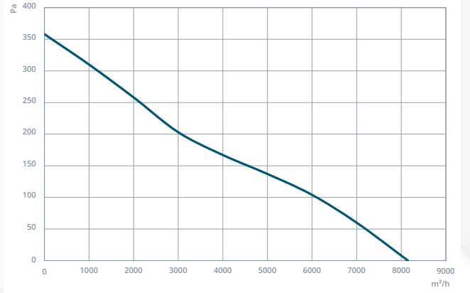
NDTF-DM 560
