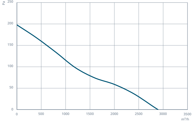
NDTF-DM 400
