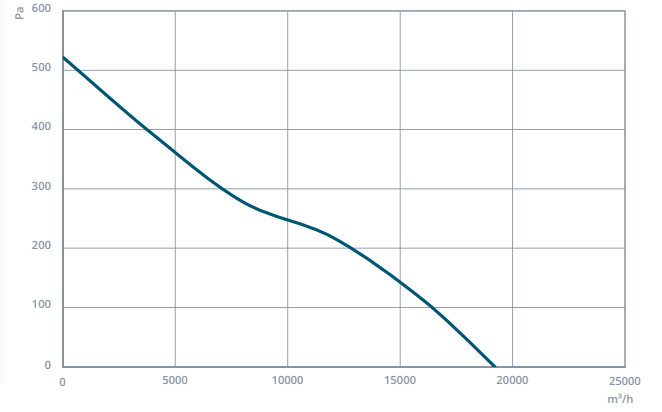
NDTF-DM 710
