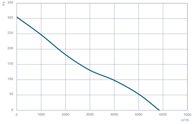
NDTF-DM 500
