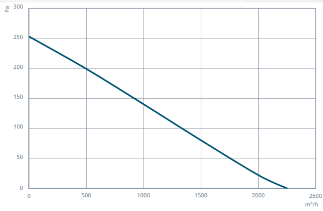
NCF3 450-5-25
