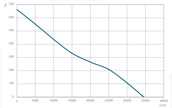
NCF3 900-5-35
