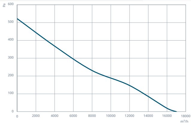
NCF3 710-5-30
