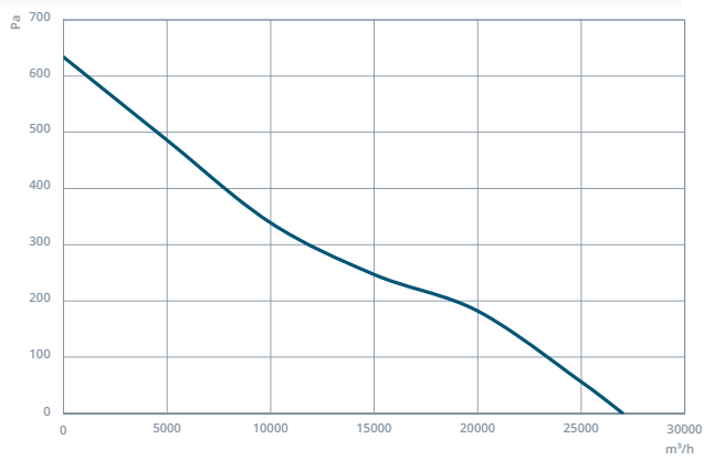
NCF3 800-5-35
