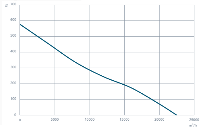
NCF3 800-5-30
