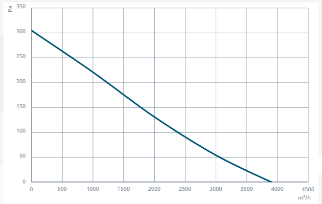
NCF3 500-5-25
